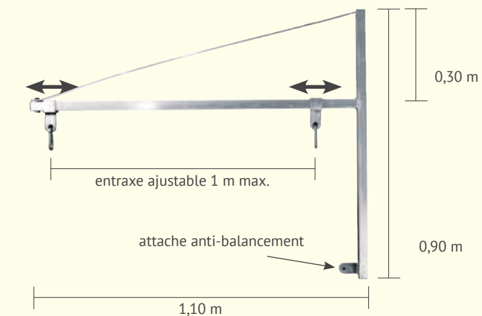
PIX01 Potence horizontale Hauteur : 0,90 m Longueur : 1,10 m Entraxe max : 1,00 m Charge maxi : 25 kg
